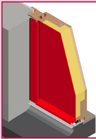
POSE EN RÉHABILITATION DANS LA FEUILLURE MAÇONNERIE
