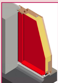
POSE EN RÉHABILITATION DANS LA FEUILLEURE MAÇONNERIE
