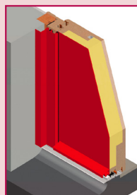
POSE EN RÉNOVATION SUR BÂTI EXISTANT
