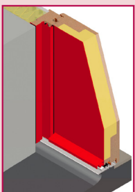
POSE EN APPLIQUE AVEC TAPÉE D'ISOLATION
