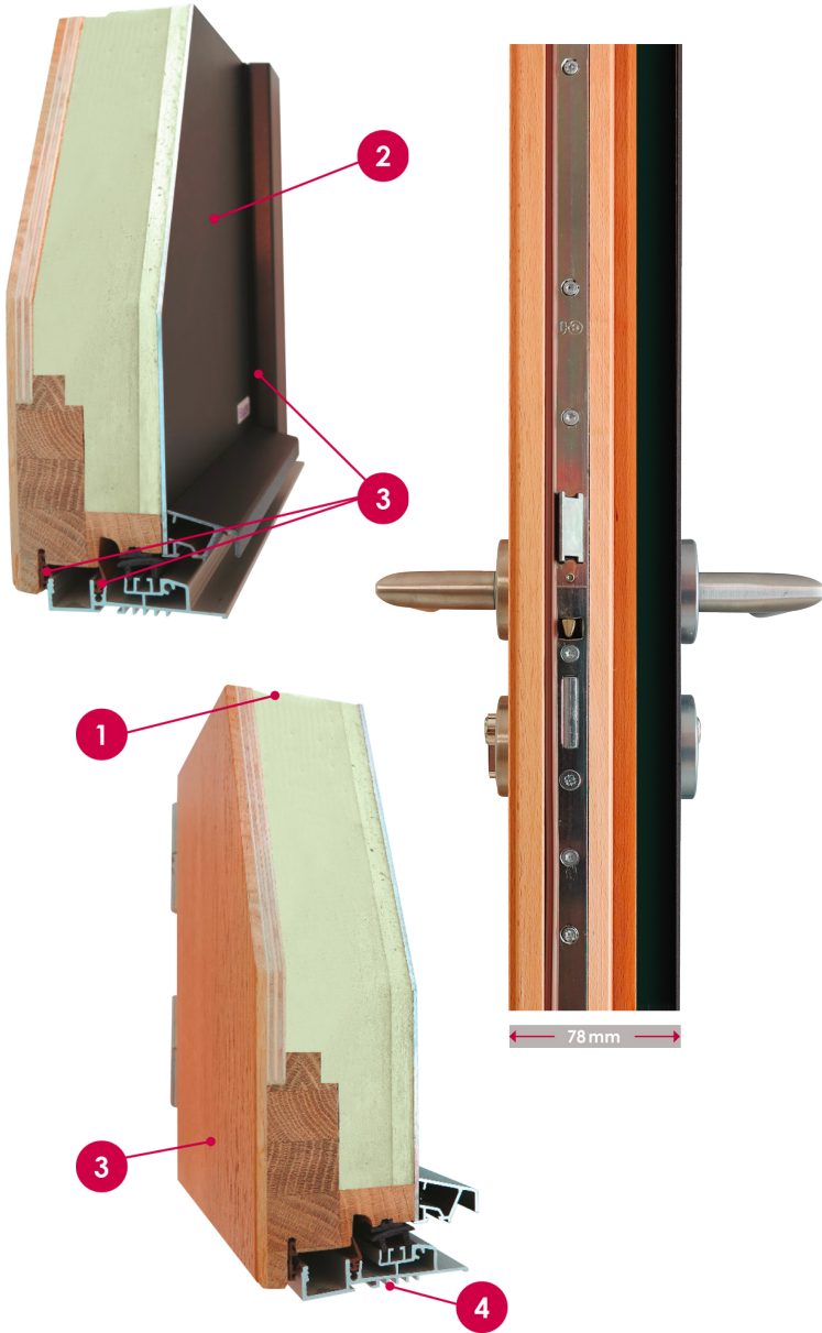
2 vantaux tiercés
